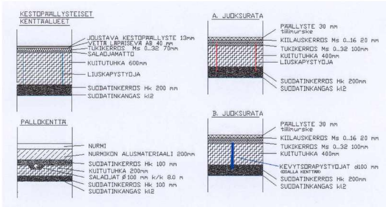
Luopioisten urheilukentälle toteutettujen rakennetyyppien poikkileikkauskuvat
